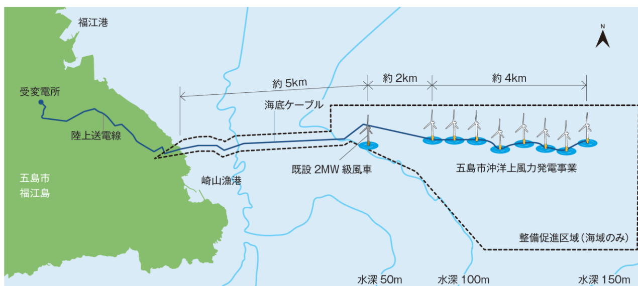
風車配置模式図
